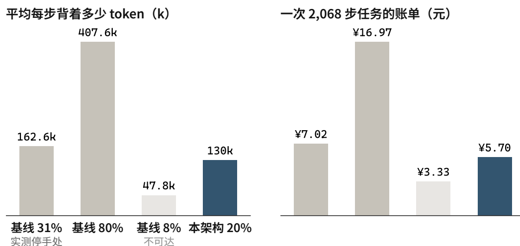
图2 三种活法与本架构的对比。31%一档是实测中人工停手的位置（中位 30.9%）；@8%一档是基线按钱算出的最优点，工程上不可达、实测里没有人能走到；本架构一档取 20% 水位、4 分支、申报 10k。数据来源：附录2 A2.4 / A2.5。
